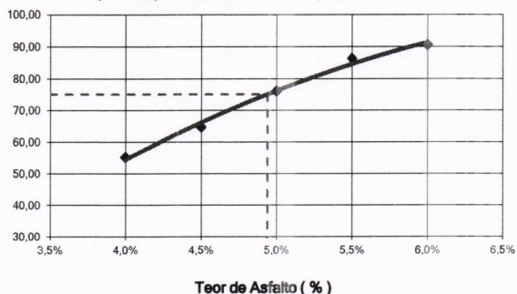
10.8) Relação Betume-Vazios (%)
